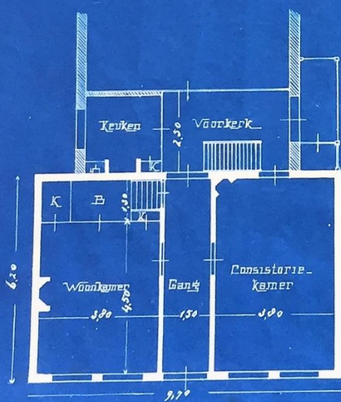
Plattegrond
